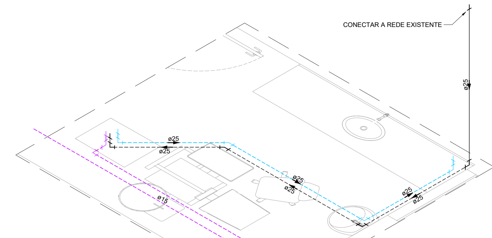
DET. HID - 1 ESCALA: 1:25
