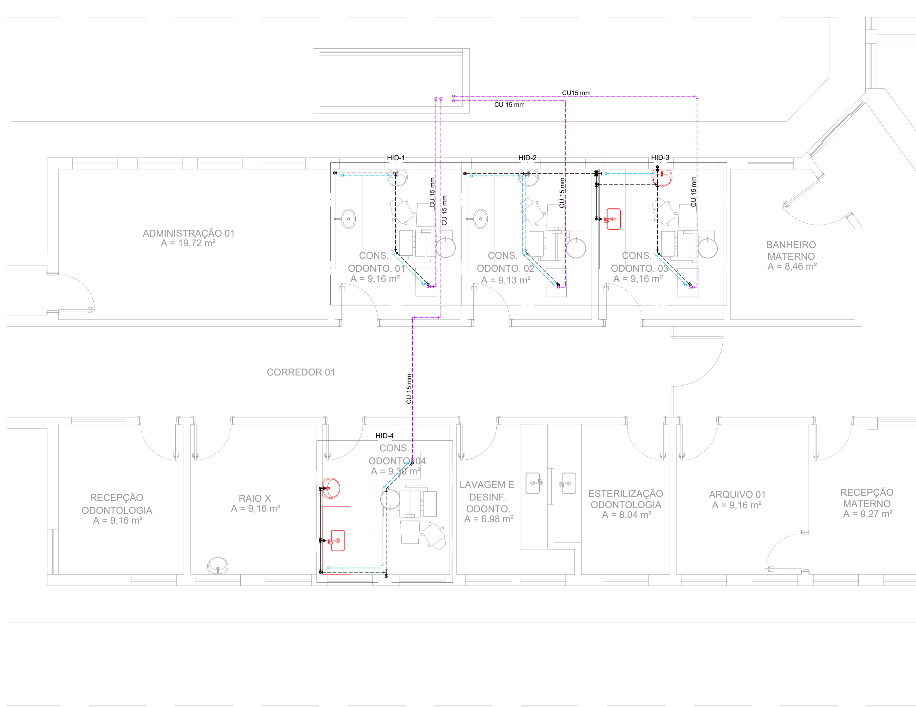
PLANTA BAIXA - TÉRREO Escala: 1:50
